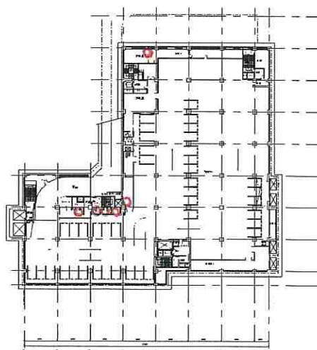
地下2階
